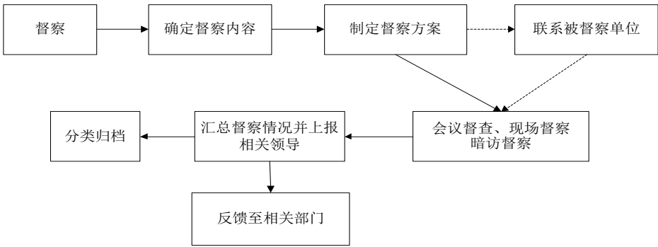
图1 督察流程图
